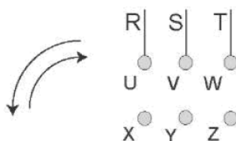
Рисунок 6. Изменение подключения для смены направления вращения электродвигателя.
