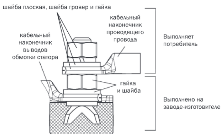
Рисунок 5. Схема контактного соединения.
